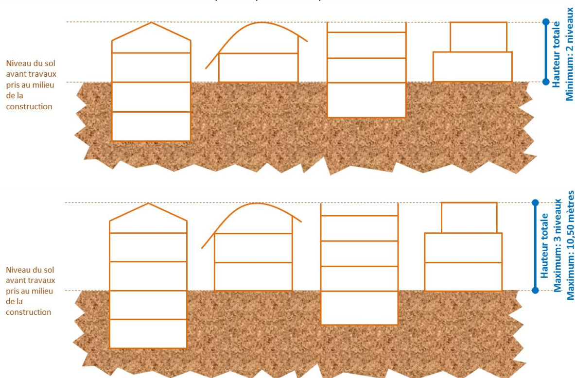
Schémas explicatifs des hauteurs minimale et maximale des constructions dans le secteur Uh
