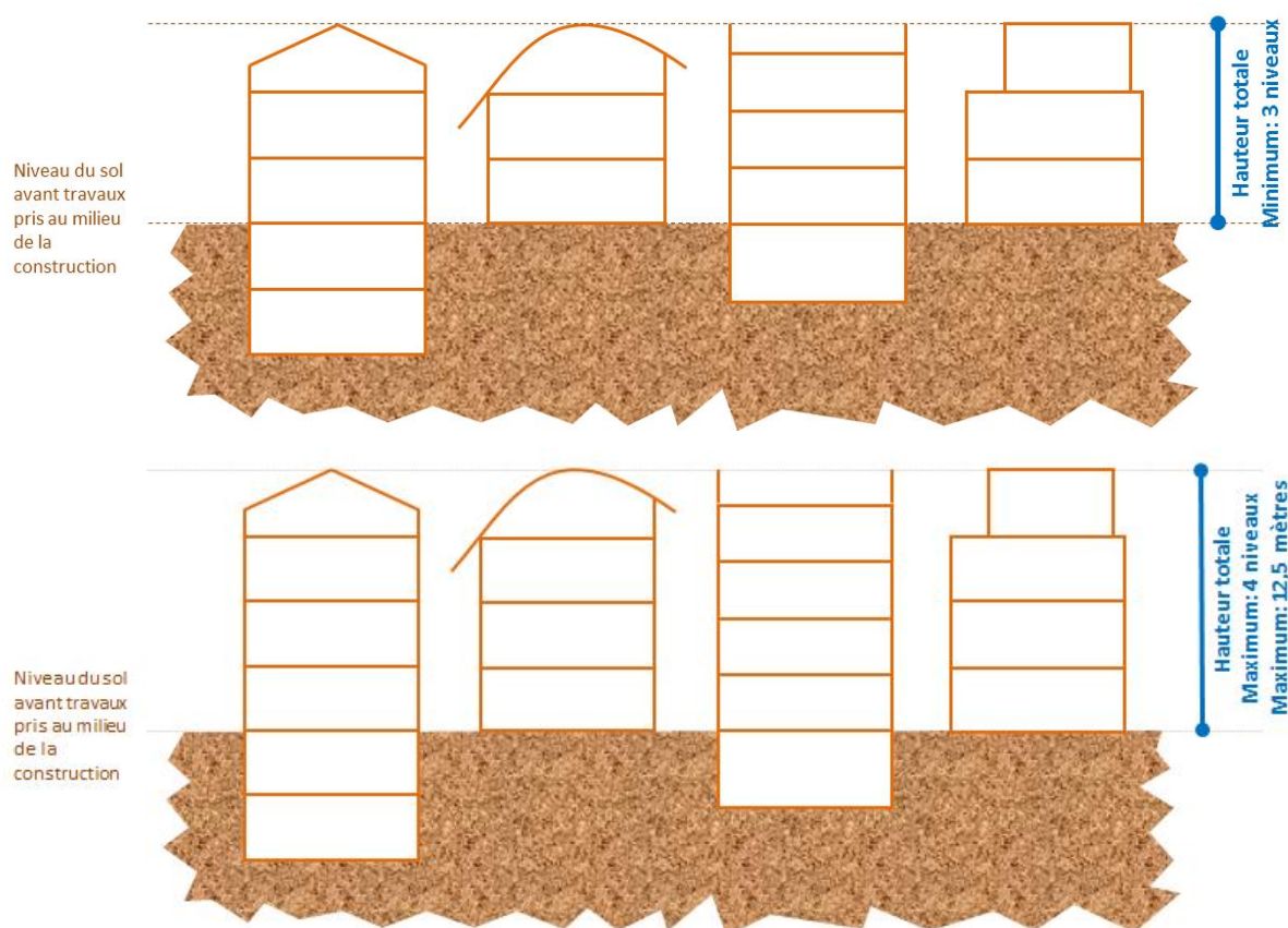
Schémas explicatifs des hauteurs minimale et maximale des constructions dans le sous-secteur 1AUsbr
